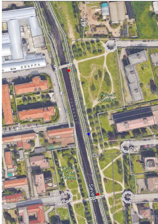
● Ubicazione misuratori di livello ● Ubicazione datalogger a pannello solare
